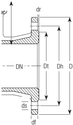
Flangeboringer iht. ISO 7005 del 2 (EN 1092-2: 1997, DIN 2501):
